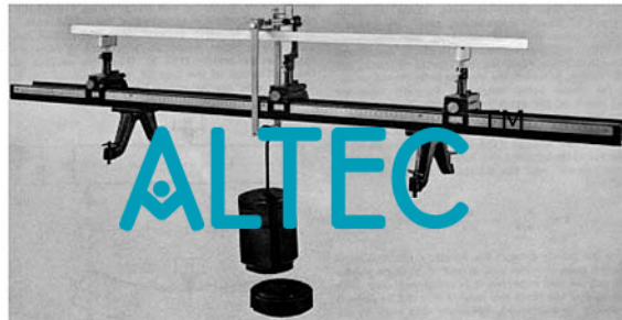
Fig. 3. Flexure Apparatus
